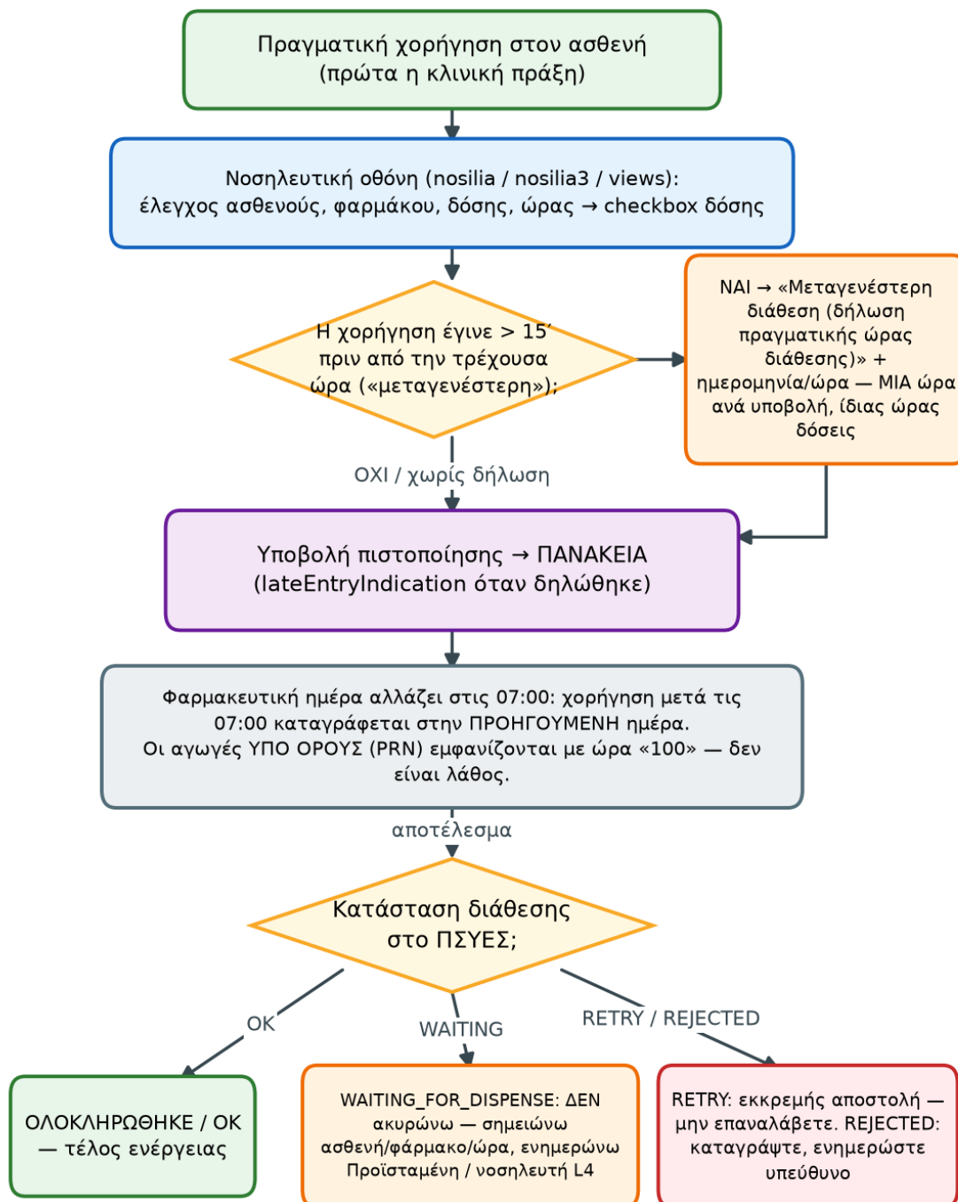
Διάγραμμα ροής: πιστοποίηση χορήγησης και ενδείξεις ΠΣΥΕΣ
